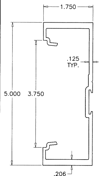
③A DOOR MULLION
