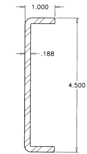
⑬ STEEL REINFORCING 36 KSI MIN.
